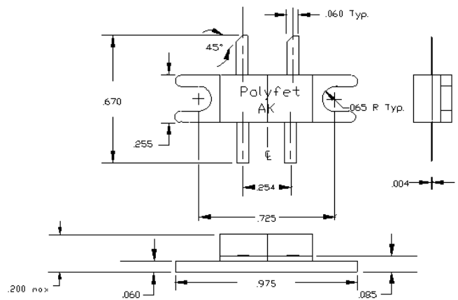
Polyfet AK Package
