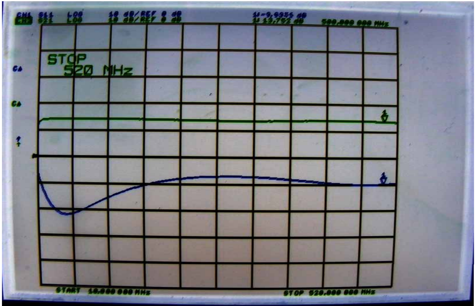
TB219#3 Vds=28Vdc, Idq=200mA, Pin=0dBm
